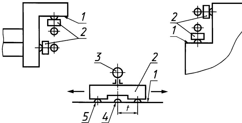
Измерение прямолинейности
