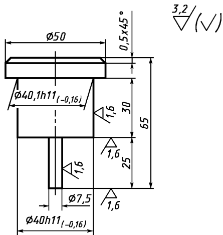
Рисунок Б.3 — Пуансон
