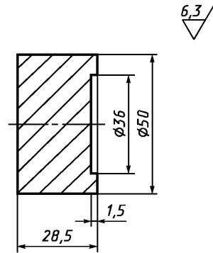
Рисунок Ж.7 — Накладка
