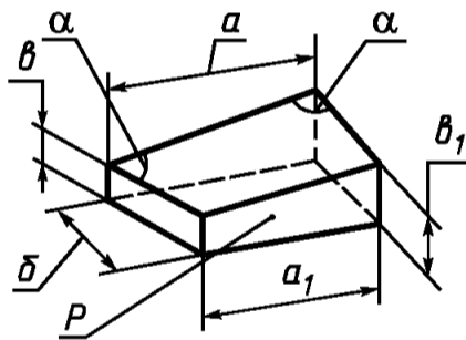
Рисунок 4 — Размеры трапецидального клина с соотношением \frac{b}{b_1} \leq 1
