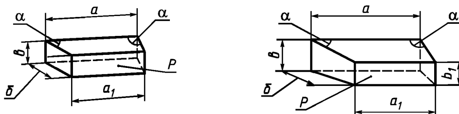
Рисунок 3 — Трапецидальный клин
