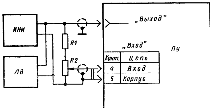
Схема для проверки нелинейных искажений
