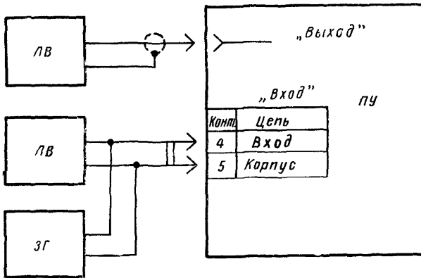
ЛВ—ламповый вольтметр, ЗГ—звуковой генератор, ПУ—прибор управления
