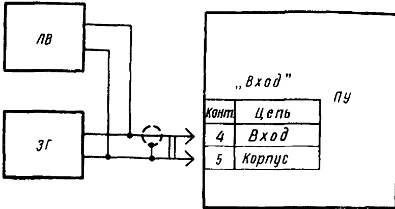
ЛВ — ламповый вольтметр; ЗГ — звуковой генератор; ПУ — прибор управления Черт. 5
