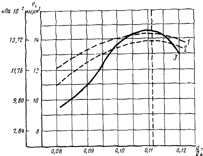
Детонационные характеристики топлив
