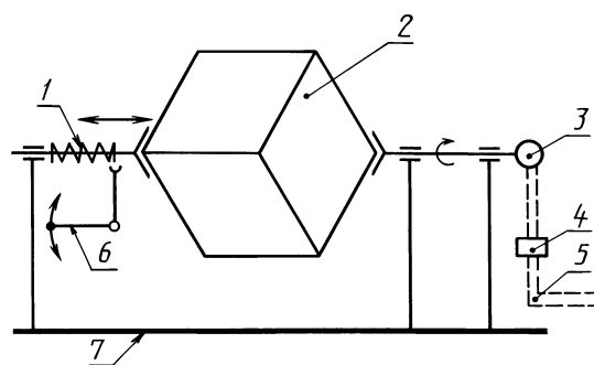
1 — пружина; 2 — куб; 3 — микроmotor; 4 — реле времени; 5 — подача энергии; 6 — рычаг; 7 — станина
