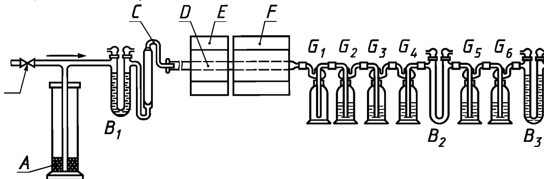
A — цилиндр с ртутью; B 1 — B 3 — U-образные трубки; C — реометр; D — трубка из кварца; E — электропечь, обеспечивающая температуру нагрева 800—900 °С; F — электропечь, обеспечивающая температуру нагрева 400—450 °С; G 1 — G 6 — склянки Дрекселя
