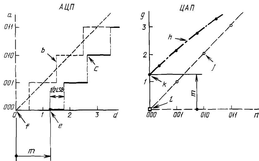
а) Смещение (указано для ступени 000)
