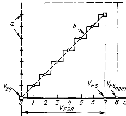
а) Однополярный АЦП
