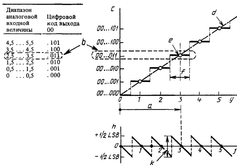
а) Идеальный линейный АЦП
