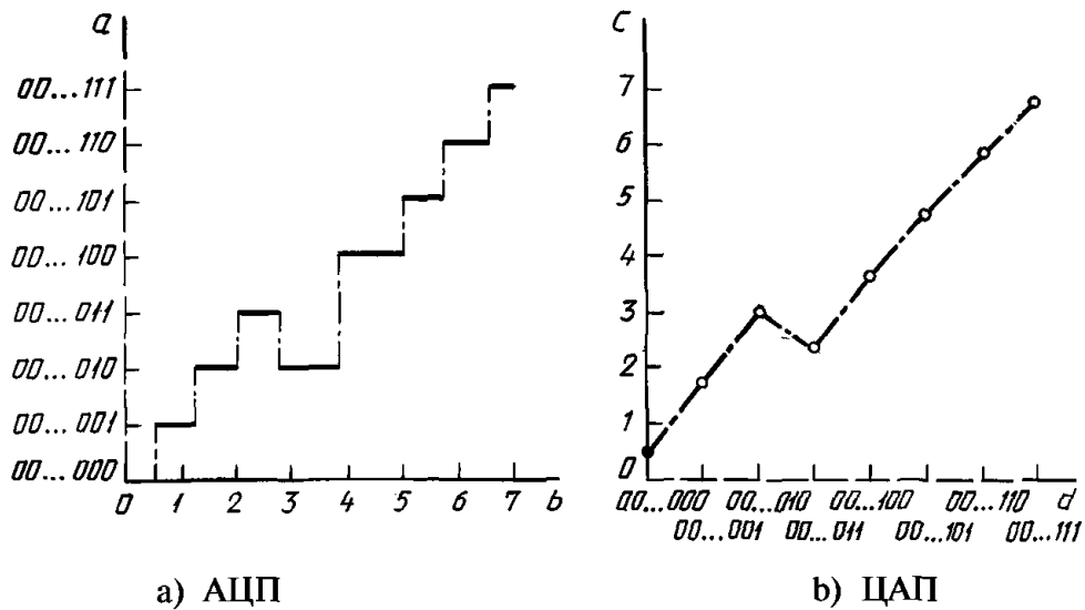
a — цифровые выходные коды; b — аналоговые входные величины (LSB); c — аналоговые выходные величины (LSB); d — цифровые входные коды
