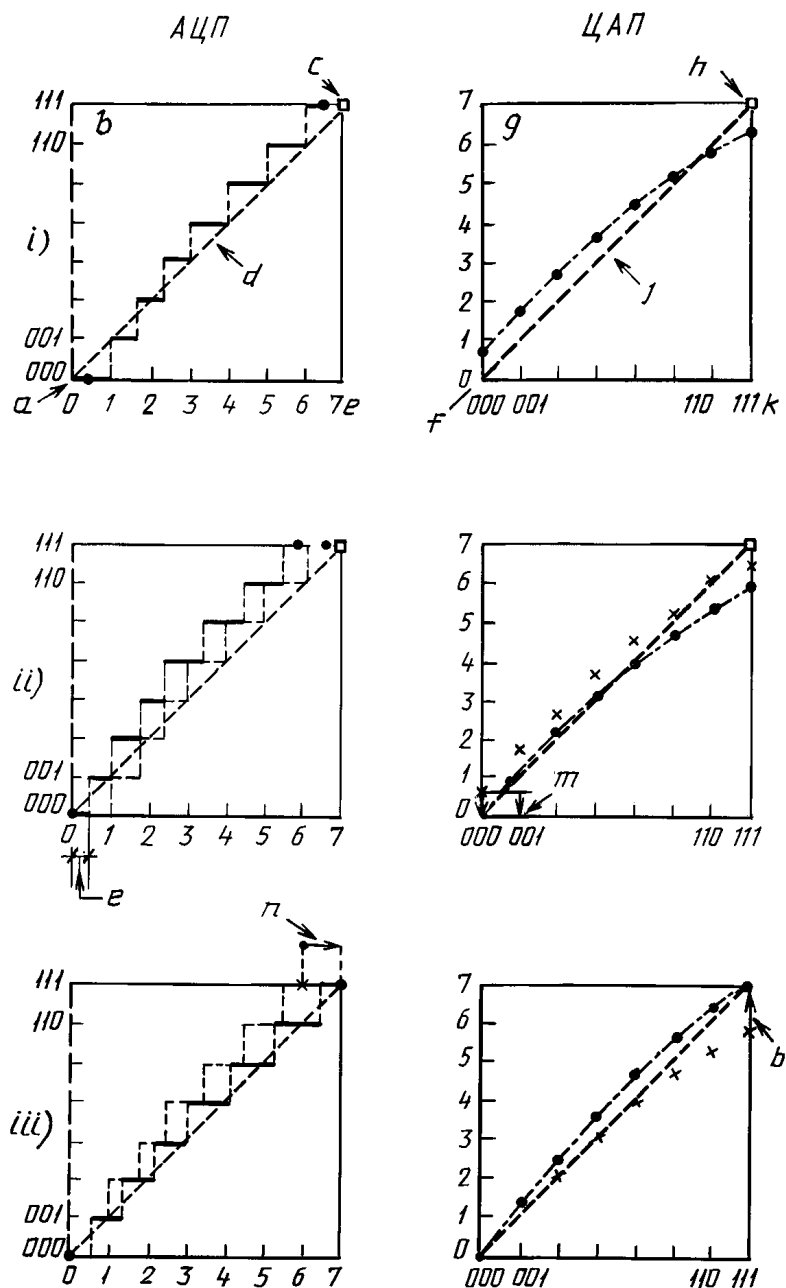
i) — до регулировки; ii) — после регулировки смещения; iii) — после регулировки смещения и коэффициента преобразования; a, f — точки смещения; b — цифровые выходные коды; c, h — точка наклона; d, j — идеальная прямая; e — аналоговые входные величины; g — аналоговые выходные величины; k — цифровые входные коды; l, m — регулировка смещения; n, p — регулировка коэффициента преобразования
