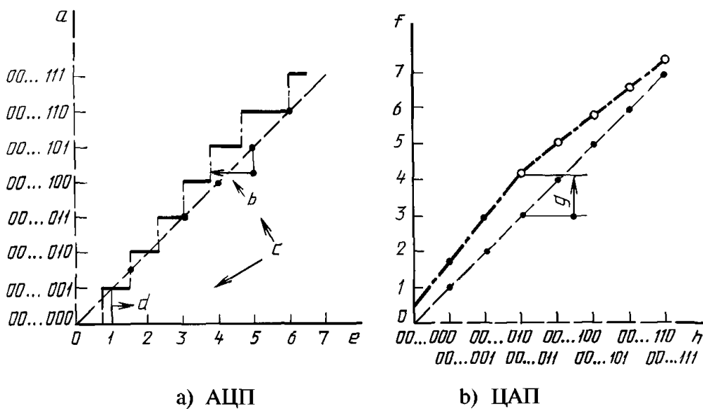
a — цифровые выходные коды; b — на ступени 00...101 ( -1 \frac{1}{4} LSB); c — полная погрешность; d — на ступени 00...001 ( + \frac{1}{2} LSB); e — аналоговые входные величины (LSB); f — аналоговые выходные величины (LSB); g — общая погрешность на ступени 00...011 ( + 1 \frac{1}{8} LSB); h — цифровые входные коды
