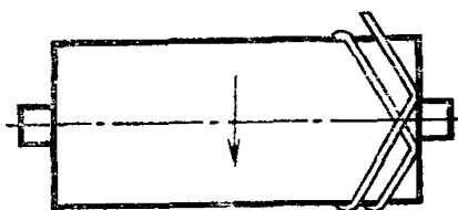
Отстающая намотка
