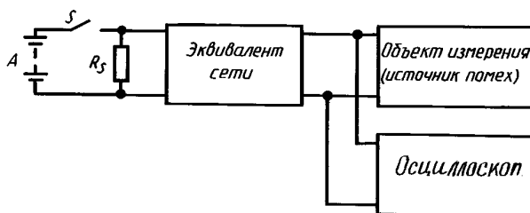
A — аккумулятор; S — мощный выключатель; R_c — нагрузочное сопротивление
