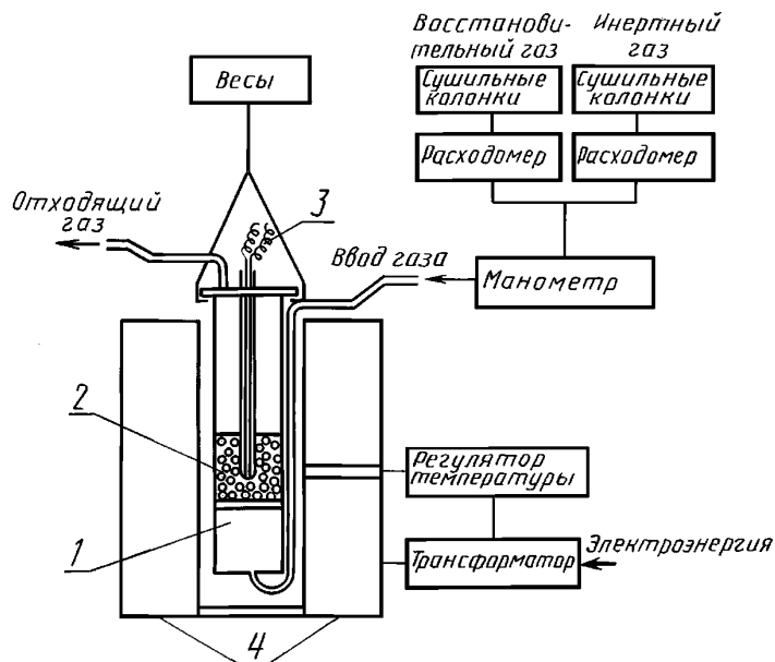
Схема аппарата для проведения исследования восстановимости
