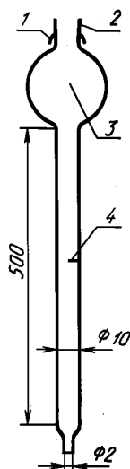
Стеклянная адсорбционная колонка вместимостью 50 см 3
