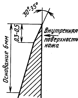
Рекомендуемая режущая кромка
