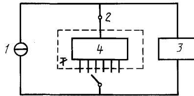
1 — генератор постоянного тока; 2 — контрольная точка; 3 — пороговый детектор; 4 — испытуемый прибор Черт. 2
