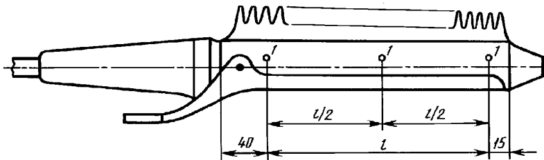
Схема прикрепления термодатчиков на электрощипцах и электрорасческах
