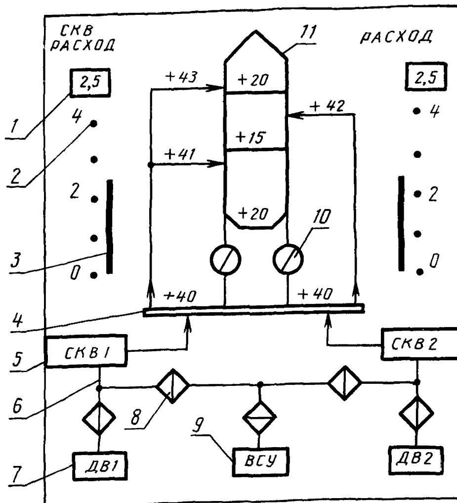
1 — счетчик; 2 — отметки шкалы указателя расхода воздуха; 3 — указатель расхода воздуха; 4 — коллектор; 5 — система кондиционирования воздуха; 6 — магистрали отбора воздуха от двигателя; 7 — двигатель 1; 8 — кран кольцевания; 9 — вспомогательная силовая установка; 10 — вентилятор; 11 — контур кабины; +15, +20, +40, +41, +42, +43 — значения температуры в коллекторе, трубопроводах, салонах; 0, 2, 4 — оцифровка шкалы указателя расхода воздуха
