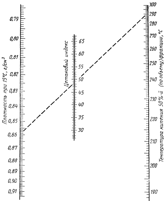
Номограмма для определения цетанового индекса (ЦИ)
