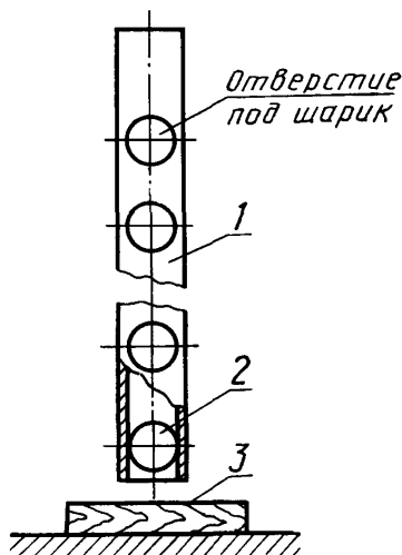
1 — направляющая труба; 2 — шарик; 3 — испытуемый образец
