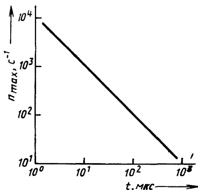
n — максимальная скорость счета импульсов; t — разрешаемое время блока обработки данных
