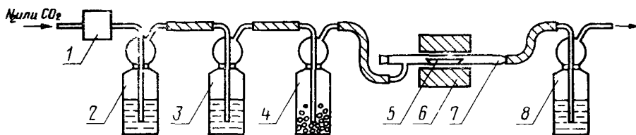
Схема установки для пиролиза
