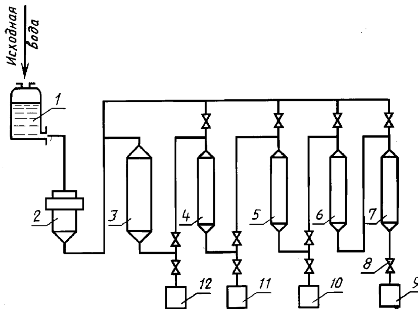
Схема лабораторной установки для очистки исходной воды
