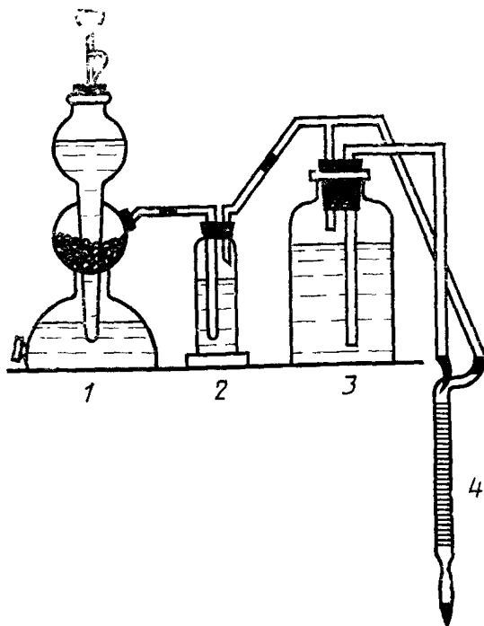
1—аппарат Киппа; 2—промывалка для газа, заполненная раствором сернистого титана (III) 50 г/дм 3 ; 3—сосуд с рабочим раствором, 4—бюретка.
