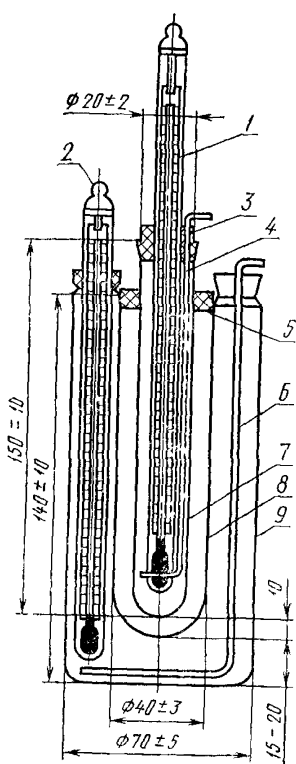
1 — специальный термометр, 2 — термометр, 3, 5 — пробки, 4, 6 — мешалки, 7 — пробирка, 8 — впаиваемая пробирка, 9 — стакан
