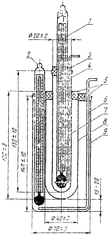
1 — специальный термометр, 2 — термометр; 3, 5 — пробки, 4, 6 — мешалки, 7, 8 — пробирки, 9 — стакан
