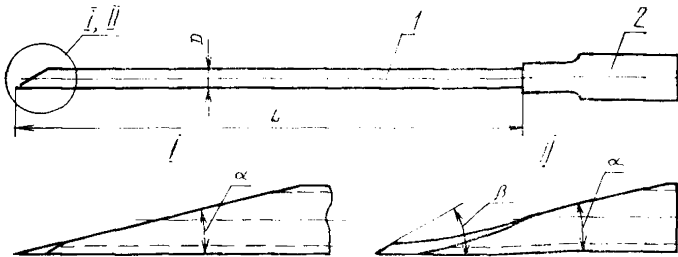
1—головка; 2—труба Черт. 1
