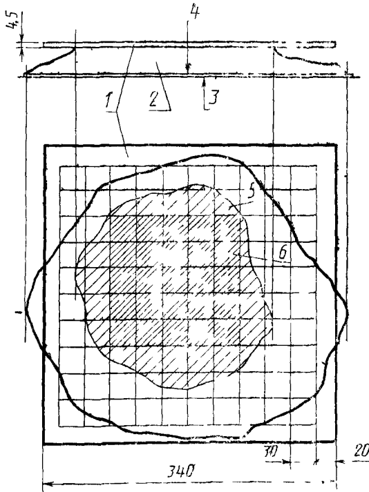
1 — лист стекла; 2 — смола, 3 — твердая плита, 4 — лист глянцевой белой бумаги, 5 — участок контакта между стеклом и смолой; 6 — 25 квадратов, выбранных для подсчета
