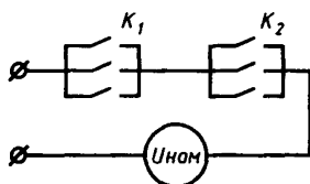
K_1 — K_2 —контакты главной цепи пускателя; U_{ном} —индикатор
