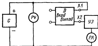
G —генератор постоянного тока; PV —измеритель напряжения; D —измеряемый прибор; X1, X2 —контакты подключения измеряемого прибора; УЗ —устройство защиты измеряемого прибора от перегрузки при коротком замыкании; РА —измеритель тока
