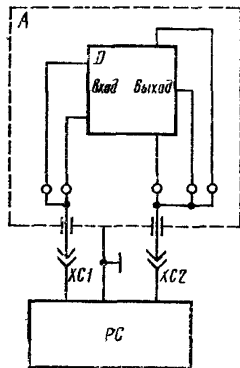
A —устройство подключения; D —измеряемый прибор; XC1 , XC2 —разъемное соединение устройства подключения и измерителя емкости; РС —измеритель емкости
