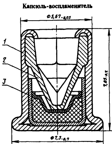
1 — оболочка; 2 — наковальня; 3 — малый капсюль-воспламенитель
