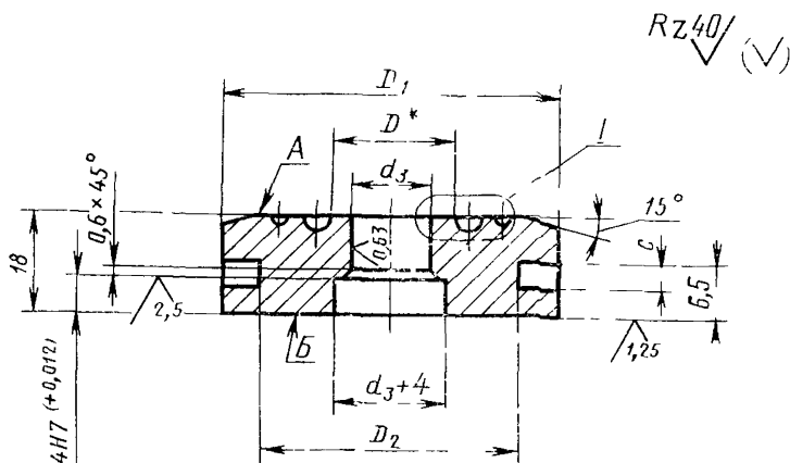
Матрица (поз. 1)
