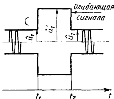
Форма сигнала на входе усилителя
