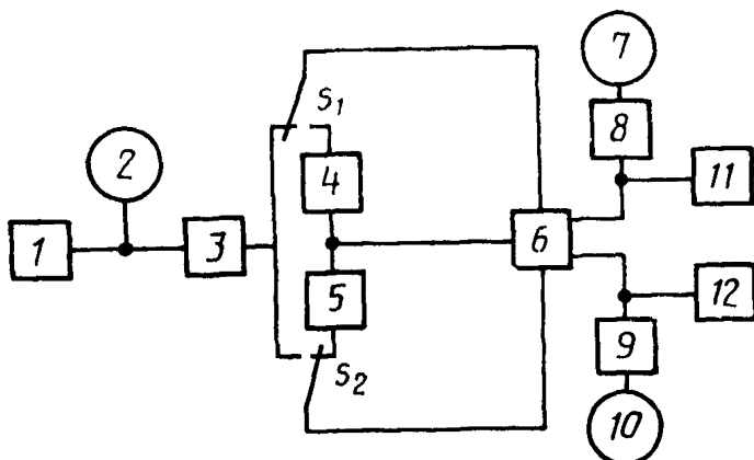
1 — генератор; 2, 7, 10 — вольтметры; 3 — согласующее звено, 4, 5 — эквиваленты сопротивления источника; 6 — измеряемый усилитель; 8, 9 — фильтры; 11, 12 — эквиваленты нагрузки; S_1, S_2 — переключатели
