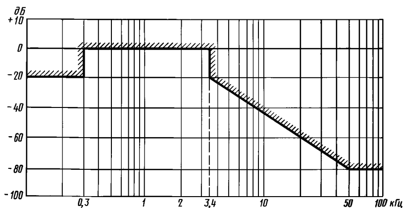
Нормированный уровень мощности спектральных составляющих факсимильного сигнала
