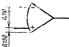
Усилитель операционный с дифференциальным входом
