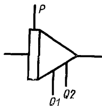
Усилитель интегрирующий
