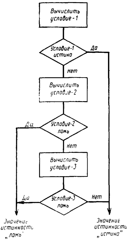
Рис. 3. Вычисление выражения условие-1 OR условие-2 AND условие-3 (условие-1 ИЛИ условие-2 И условие-3)
