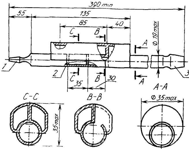
1 — корн шлифа А, 2 — кварцевая фритта, крупная, 3 — корн шлифа Б Черт. 2
