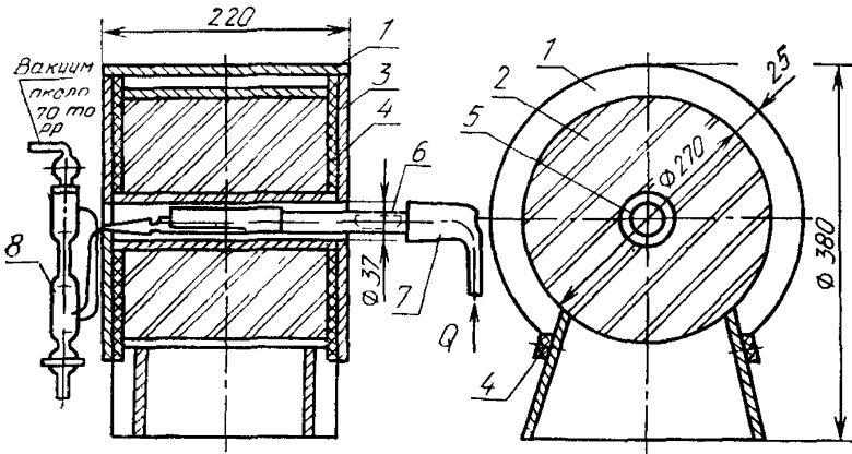
1 — алюминиевая металлическая обшивка (открыта сбоку) 2 — кизельгур, 3 — алюминиевый боковой лист, 4 — асбест, 5 — керамическая трубка; 6 — кварцевая трубка для сжигания; 7 — форштос; 8 — абсорбционный сборник Черт. 1
