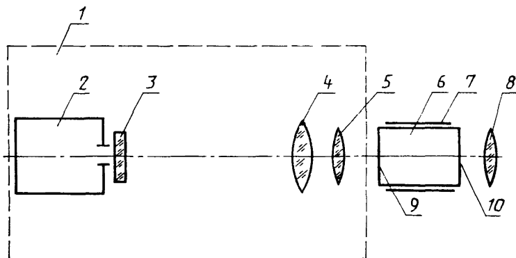
1—проектор; 2—осветитель; 3—мира; 4—коллимационный объектив; 5—проекционный объектив; 6—ЭОП; 7—держатель ЭОП; 8—окулярная оптика; 9—фотокаатод; 10—экран
