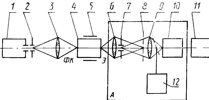
1 — осветитель; 2 — диафрагма со щелью; 3 — входная оптика (микрообъектив в обратном ходе); 4 — ЭОП; 5 — держатель ЭОП; 6 — выходной микрообъектив; 7 — выходной зрочок микрообъектива поз. 6; 8 — анализирующий растр; 9 — коллектив; 10 — приемник излучения, 11 — регистрирующее устройство; 12 — микроскоп; ФК — фотокатод; Э — экран; А — анализирующий блок
