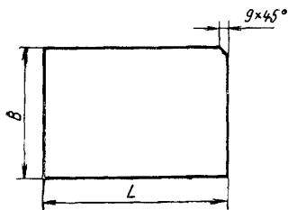
Черт. 1
