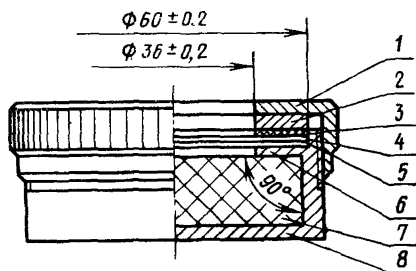
1—крышка, 2—металлическая прокладка, 3—резиновая прокладка, 4—образец, 5—влагонепроницаемая пленка, 6—заплевки, 7—вкладыш из пенополиуретана, 8—металлический стаканчик
