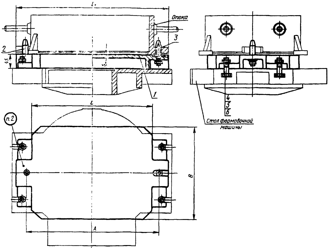
1 — плита по табл. 1; 2 — штырь центрирующий 0290-2501 по ГОСТ 20122—74 (кол. 1); 3 — штырь направляющий 0290-2551 по ГОСТ 20122—74 (кол. 1); 4 — болт М12×50,66,05 по ГОСТ 7808—70 (кол. 4); 5 — гайка М12,6,05 по ГОСТ 5927—70 (кол. 6); 6 — шайба 12,65Г,05 по ГОСТ 6402—70 (кол. 6).
