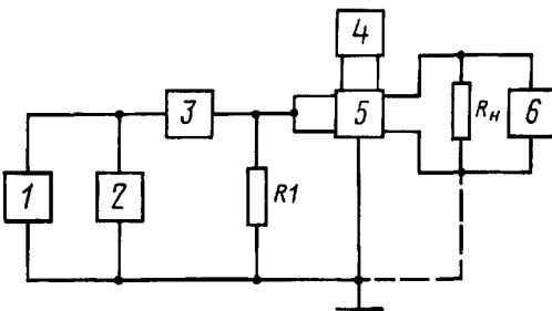
1 — генератор переменного напряжения; 2, 6 — измеритель переменного напряжения; 3 — аттенюатор; 4 — источник питания; 5 — микросхема
