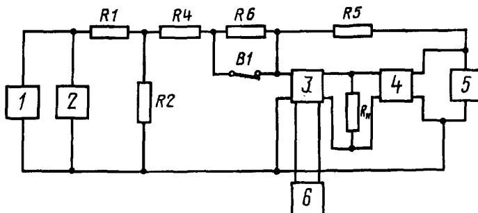
1 — источник постоянного напряжения для балансировки микросхемы; 2, 5 — измерители постоянного напряжения; 3 — микросхема; 4 — усилитель, инвертирующий фазу; 6 — источник питания
