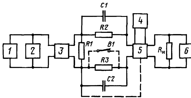
1 — генератор переменного напряжения; 2, 6 — измерители переменного напряжения; 3 — аттенюатор; 4 — источник питания; 5 — микросхема
