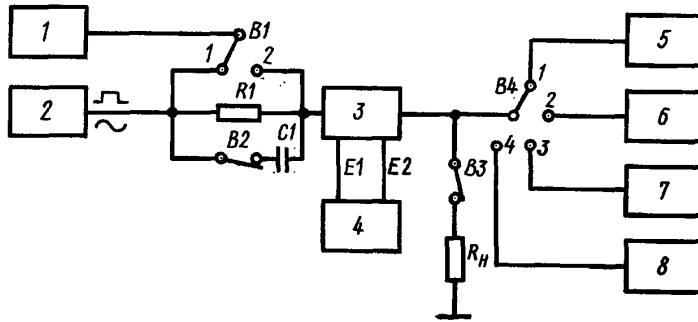
1 — измеритель переменного напряжения; 2 — генератор сигналов; 3 — микросхема; 4 — источник питания; 5 — измеритель временных интервалов; (осциллограф); 6 — измеритель переменного напряжения; 7 — измеритель частоты; 8 — измеритель нелинейных искажений
