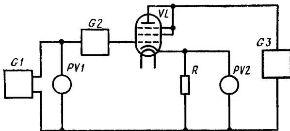
PV1 и PV2 —электронные импульсные вольтметры; G1 —генератор импульсного напряжения; R —резистор; VL —испытываемая лампа; G2 , G3 —источники напряжения постоянного тока.
