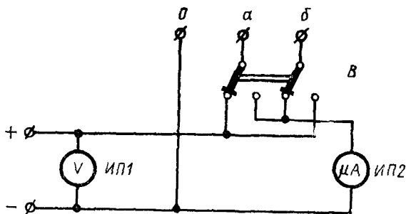
ИП1 — вольтметр постоянного тока; B — переключатель полярности напряжения; a и б — контакты, предназначенные для присоединения электродов, металлического баллона или подогревателя, между которыми измеряют сопротивление изоляции, 0 — контакт, являющийся общей точкой схемы; ИП2 — электронный или магнитоэлектрический микроамперметр постоянного тока.
