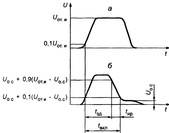
a — форма напряжения на выходе генератора G1 при отсутствии испытуемого тиристора; b — форма напряжения на испытуемом тиристоре; U_{о.с} — постоянное напряжение в открытом состоянии тиристора; U_{от.и} — импульсное отпирающее напряжение тиристора
