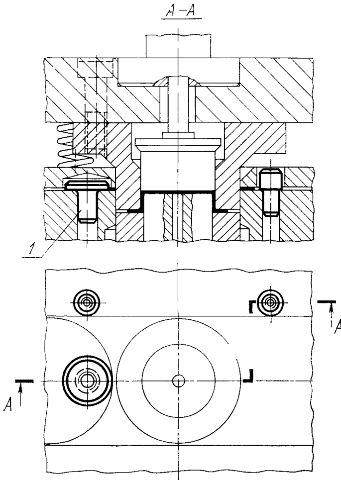
1—упор грибовый по ГОСТ 18743—80
