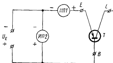
ИП1 —измеритель постоянного тока, ИП2 —измеритель постоянного напряжения, U_E —напряжение источника питания эмиттера, T —испытуемый транзистор
