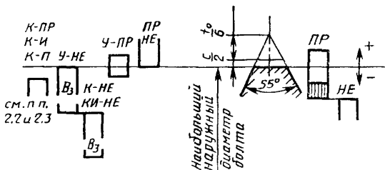
Калибры для контроля болтов (наружной резьбы)
