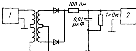
1—испытуемый диктофон; 2—детонометр.
