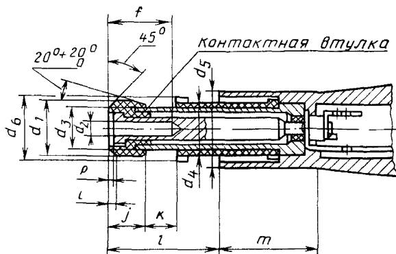
Размеры, мм
