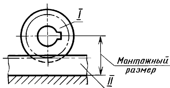
I — зубчатое колесо; II — рейка
