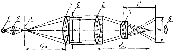
1—источник света, 2—конденсор, 3—щель коллиматора, 4—объектив коллиматора; 5—диафрагма с набором пар щелей; 6—испытуемый объектив, 7—объектив зрительной трубы, 8—окуляр микрометра
