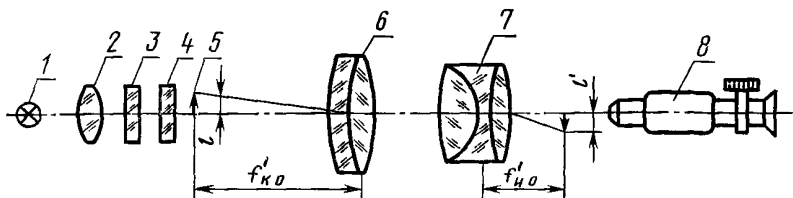
1—источник света; 2—конденсор; 3—молочное (опаловое) стекло; 4—светофильтр; 5—штриховая шкала, 6—объектив коллиматора; 7—испытуемый объектив; 8—микроскоп с окуляр-микрометром или микрометрическим поперечным перемещением
